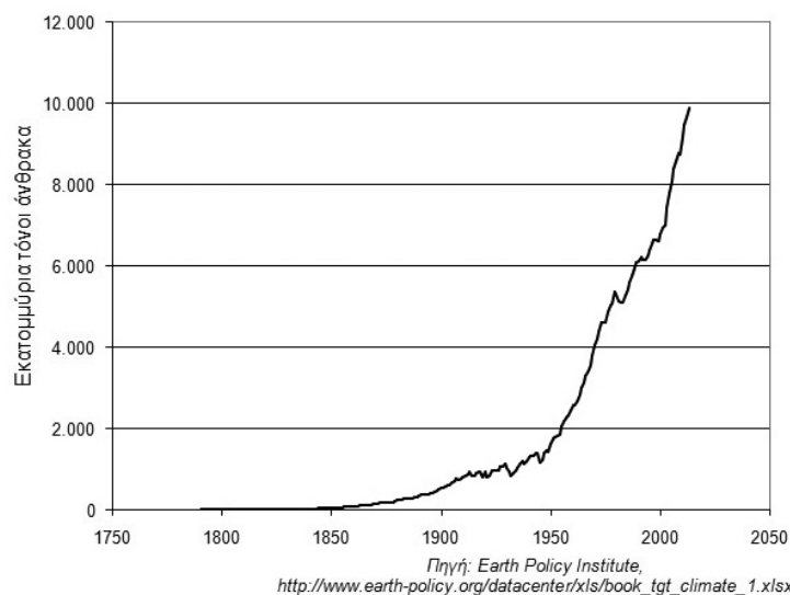
Εκπομπές διοξειδίου του άνθρακα παγκοσμίως από την καύση ορυκτών καυσίμων 1751 - 2013
